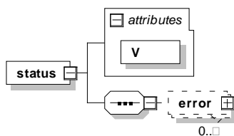
Abbildung 42: Aufbau und Kind-Elemente des Elements status
