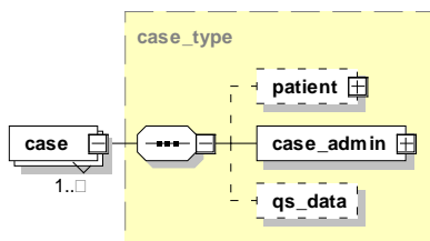
Abbildung 43: Aufbau des Elements case
