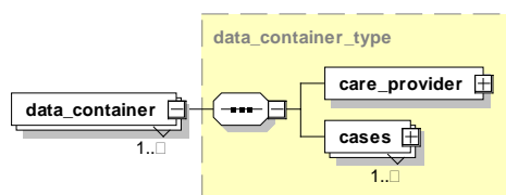
Abbildung 39: Aufbau des Elements body/data_container
