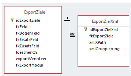
Abbildung 20: Beziehungen der administrativen Objekte – Mapping-Informationen
