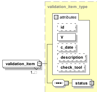
Abbildung 48: Aufbau und Kind-Elemente des Elements validation_item
