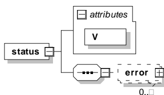
Abbildung 50: Aufbau und Kind-Elemente des Elements status
