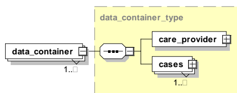
Abbildung 54: Aufbau des Elements body/data_container
