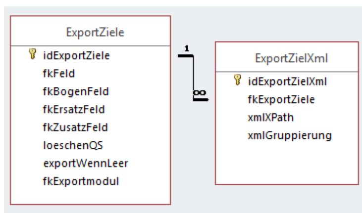
Abbildung 32: Beziehungen der administrativen Objekte – Mapping-Informationen
