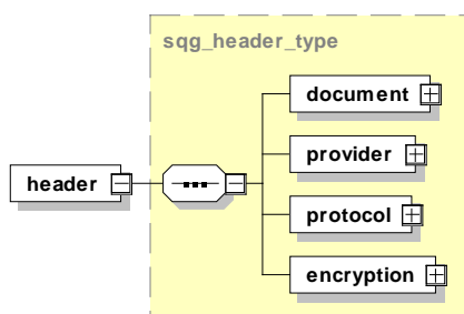
Abbildung 41: Aufbau des Elements header
