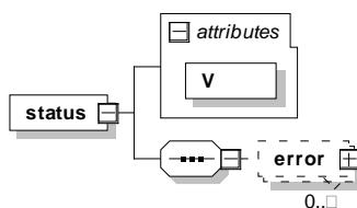
Abbildung 50: Aufbau und Kind-Elemente des Elements status
