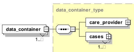
Abbildung 54: Aufbau des Elements body/data_container
