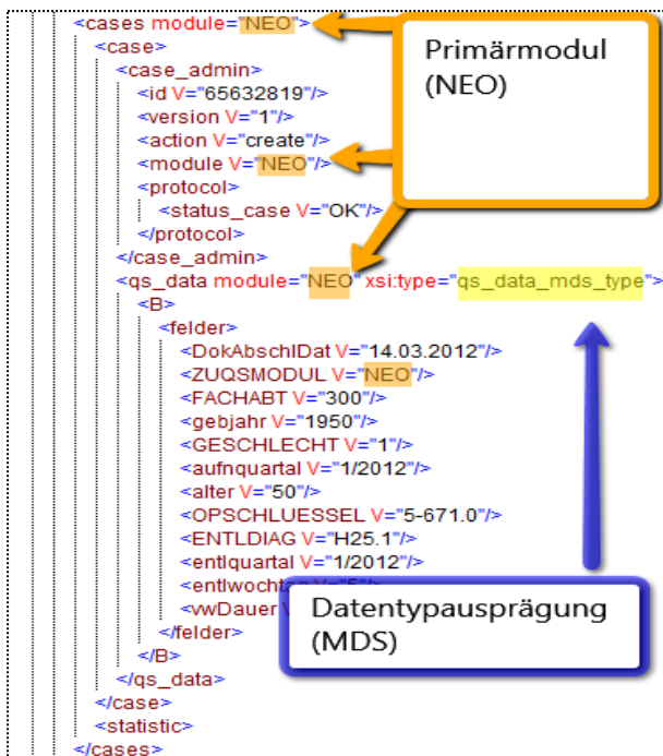
Abbildung 68: Integration des MDS in das Primärmodul
