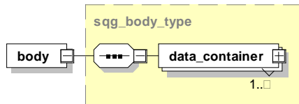
Abbildung 53: Aufbau des Elements body
