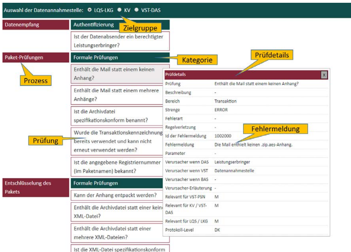
Abbildung 38: HTML-Ansicht der Prüfschritte innerhalb der QS-Dokumentation
