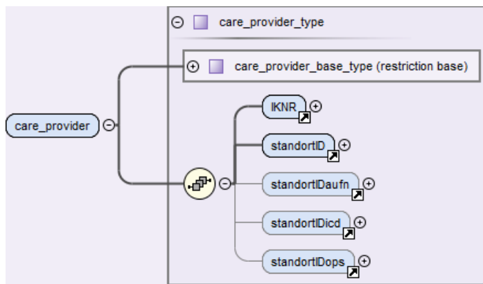
Abbildung 55: Aufbau des Elements care_provider – kollektiv-, selektivvertraglich
