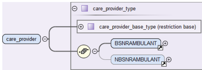
Abbildung 55: Aufbau des Elements care_provider – kollektiv-, selektivvertraglich
