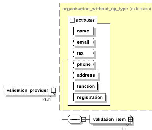
Abbildung 47: Aufbau und Kind-Elemente des Elements validation_provider
