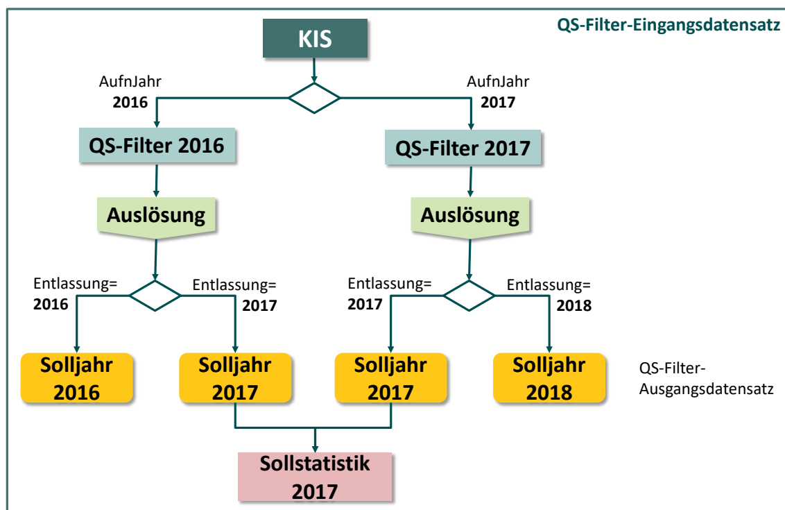
Abbildung 12: Vorgehensweise beim Erstellen der Sollstatistik für stationäre Fälle
