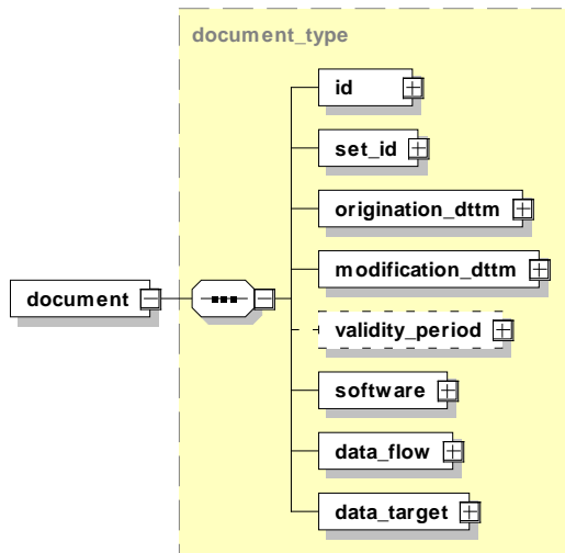
Abbildung 42: Aufbau des Elements document
