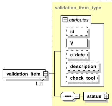
Abbildung 48: Aufbau und Kind-Elemente des Elements validation_item
