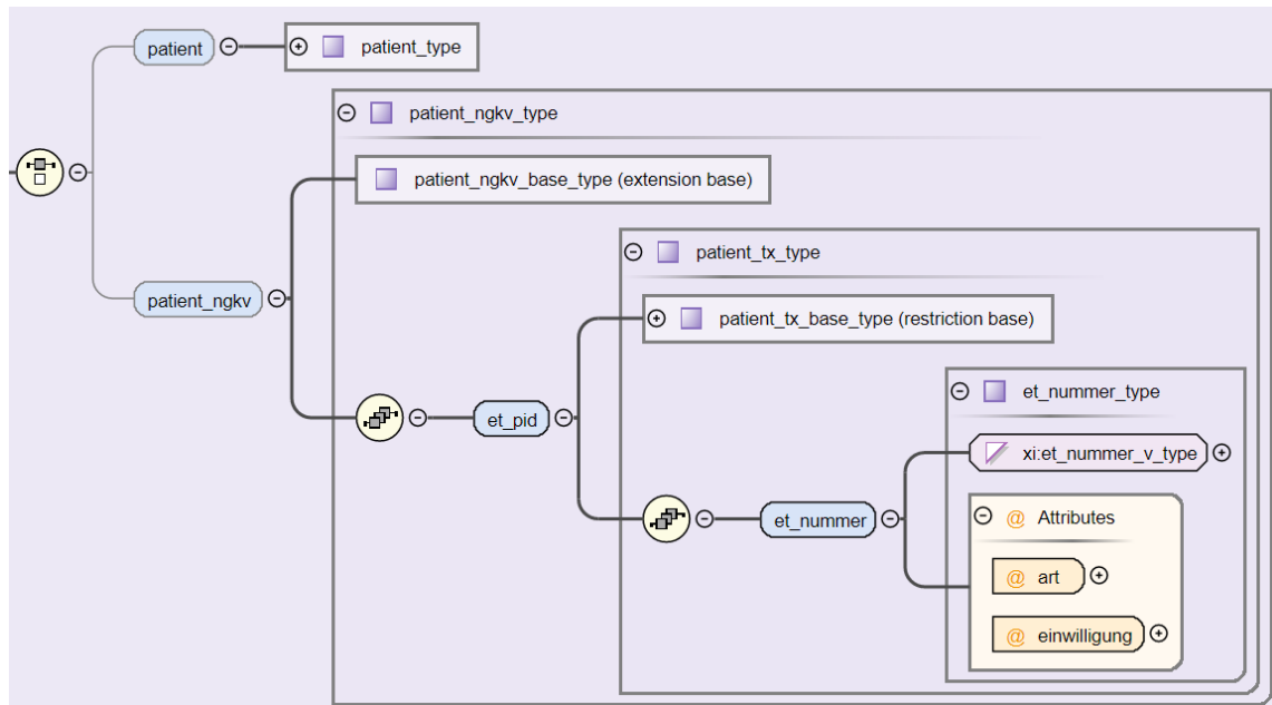
Abbildung 62: Aufbau des Elements patient_ngkv
