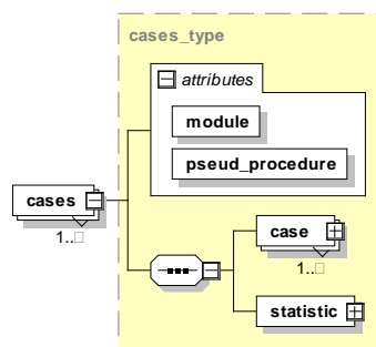
Abbildung 57: Aufbau des Elements cases
