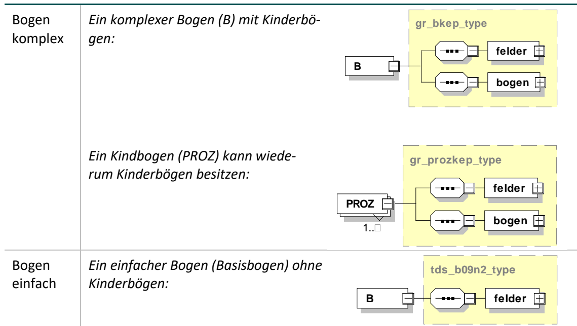
Abbildung 69: Diagramme „Bogen komplex“ und „Bogen einfach“
