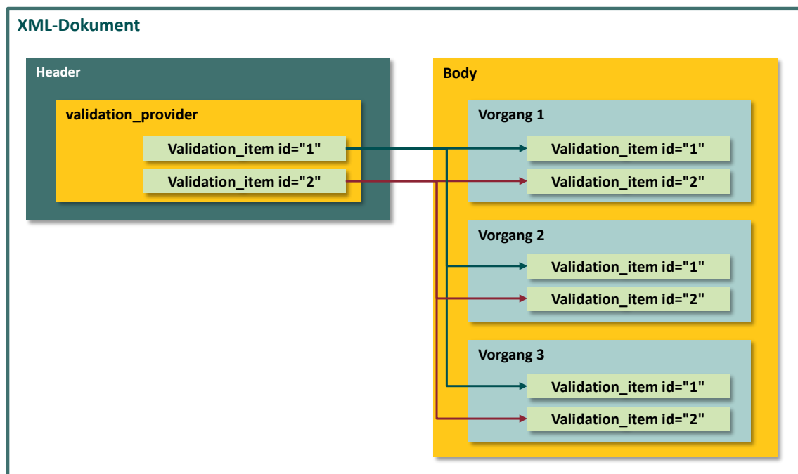
Abbildung 22: Beziehungen zwischen <validation_item> im header und <validation_item> im body über die id
