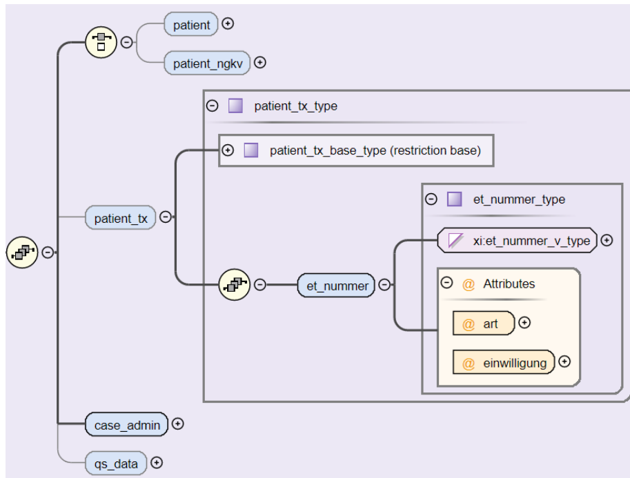
Abbildung 63: Aufbau des Elements patient_tx
