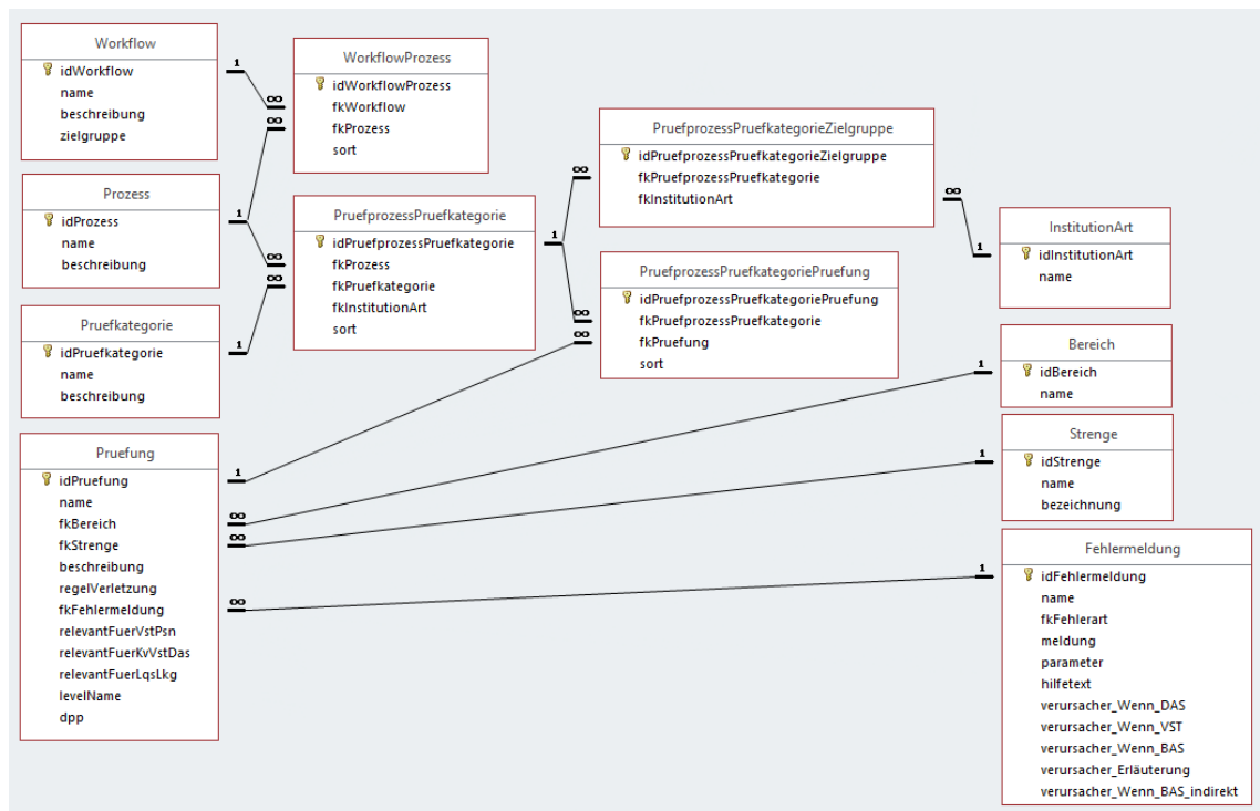
Abbildung 37: Beziehungen der administrativen Objekte – Prüfungen
