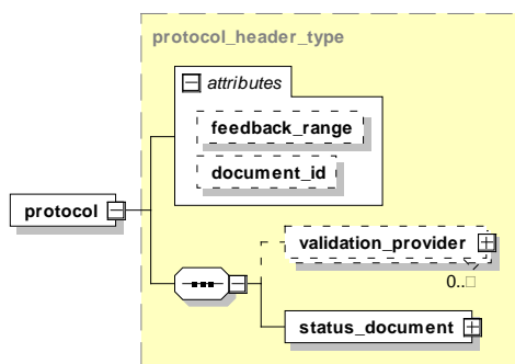
Abbildung 46: Aufbau des Elements header/protocol
