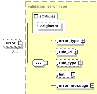
Abbildung 51: Aufbau des Elements error
