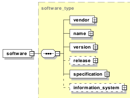
Abbildung 43: Aufbau des Elements software
