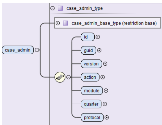
Abbildung 59: Aufbau des Elements case_admin
