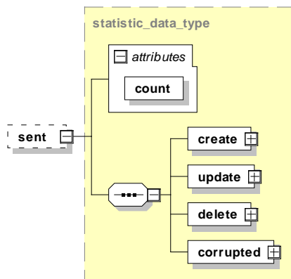
Abbildung 66: Aufbau des Elements sent
