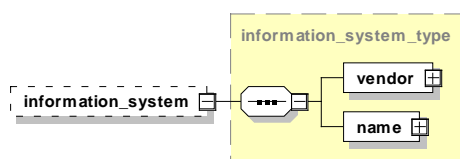
Abbildung 44: Aufbau des Elements information_system
