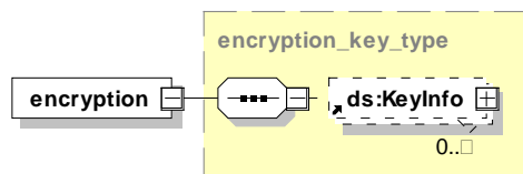
Abbildung 52: Aufbau und Attribute des Elements encryption(Krankenhaus)
