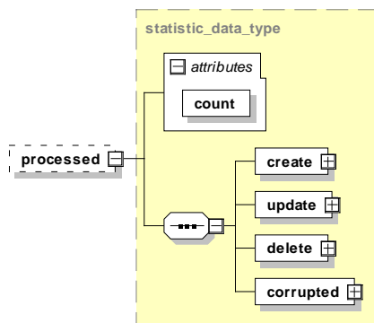
Abbildung 67: Aufbau des Elements processed
