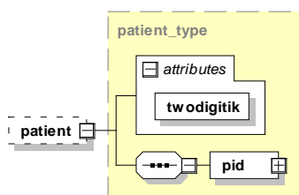
Abbildung 60: Aufbau des Elements patient
