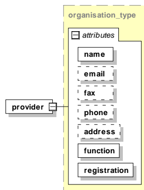
Abbildung 45: Aufbau des Elements provider
