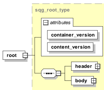
Abbildung 40: Root-Element und Kind-Elemente header und body
