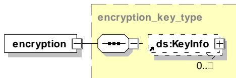
Abbildung 53: Aufbau und Attribute des Elements encryption(Krankenhaus)
