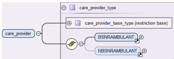
Abbildung 56: Aufbau des Elements care_provider – kollektiv-, selektivvertraglich
