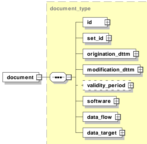
Abbildung 43: Aufbau des Elements document
