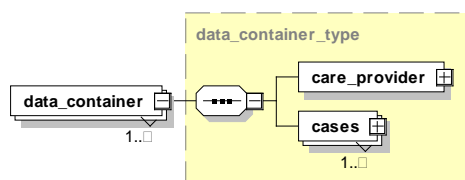
Abbildung 55: Aufbau des Elements body/data_container
