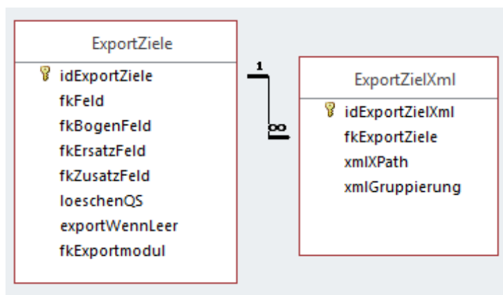
Abbildung 33: Beziehungen der administrativen Objekte – Mapping-Informationen
