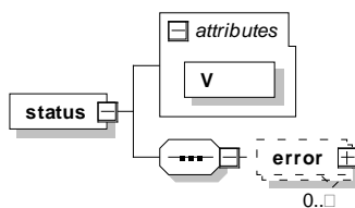
Abbildung 51: Aufbau und Kind-Elemente des Elements status
