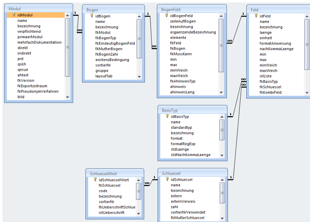
Abbildung 16: Tabellen und Relationen der Datenfeldbeschreibung (Beispiel Spezifikation 2017)
