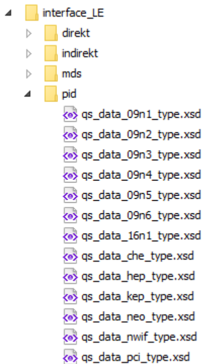
Abbildung 60: Ausprägungen des qs_data -Elements (Erfassungsmodule)
