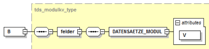
Abbildung 61: Sollstatistik-Modul
