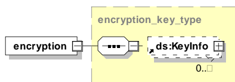
Abbildung 40: Aufbau und Attribute des Elements encryption(Krankenhaus)
