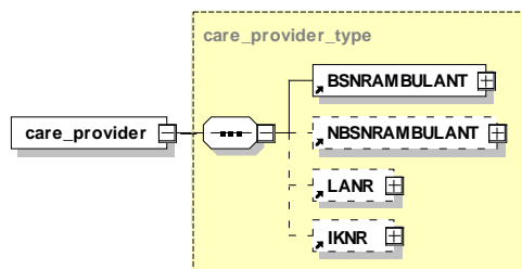
Abbildung 50: Aufbau des Elements care_provider – kollektiv-, selektivvertraglich
