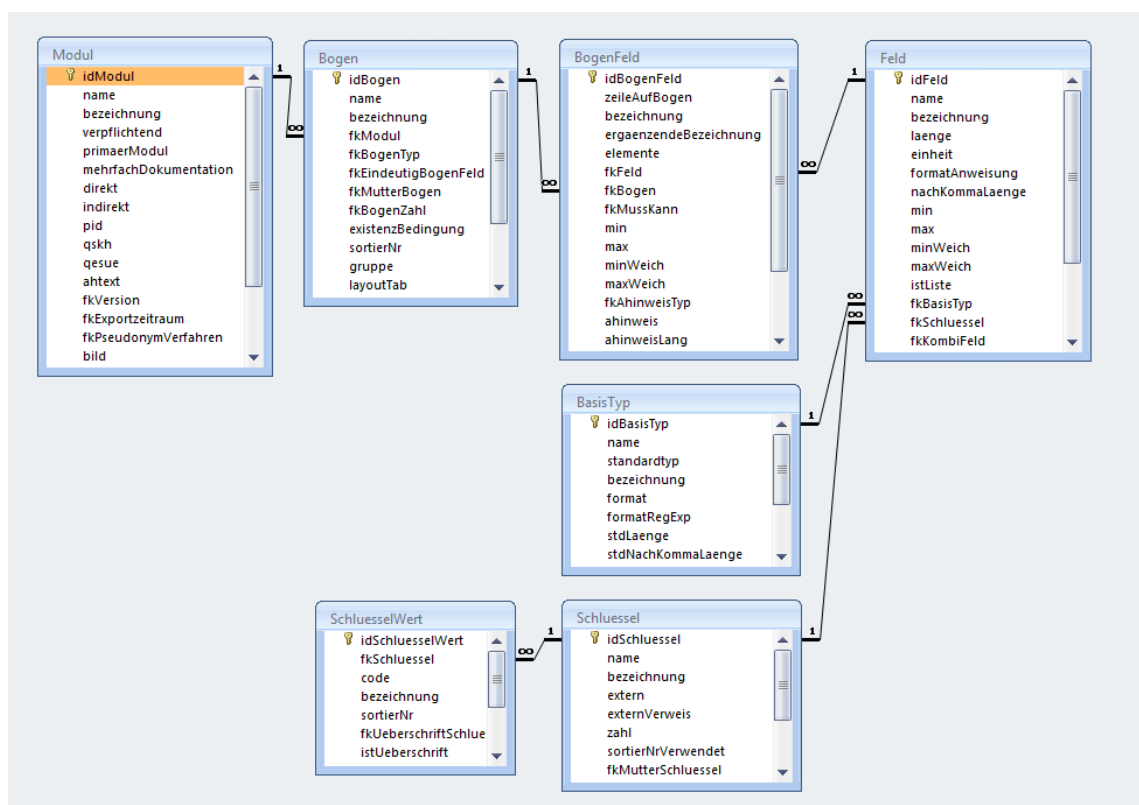
Abbildung 20: Tabellen und Relationen der Datenfelddescription
