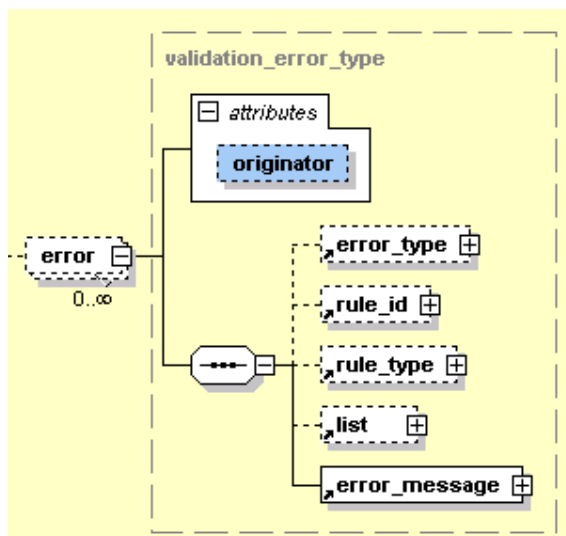
Abbildung 14: Attribut „originator“ im Prüfungs- und Fehlerprotokoll
