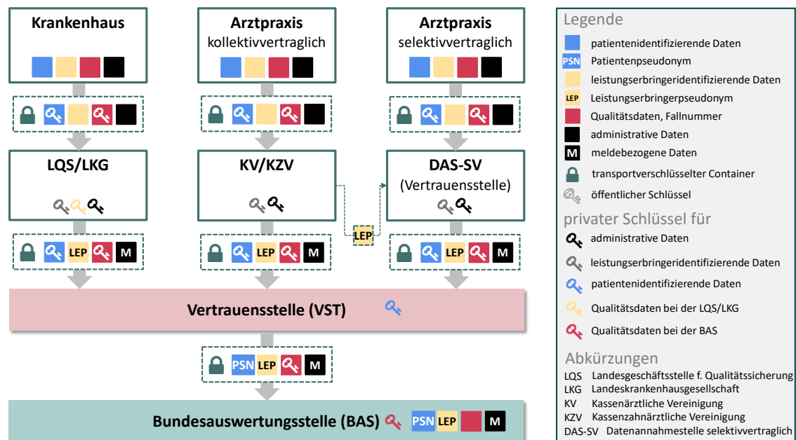
Abbildung 2: Serielles Datenflussmodell für die einrichtungs- und sektorenübergreifende Qualitätssicherung
