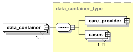
Abbildung 49: Aufbau des Elements body/data_container
