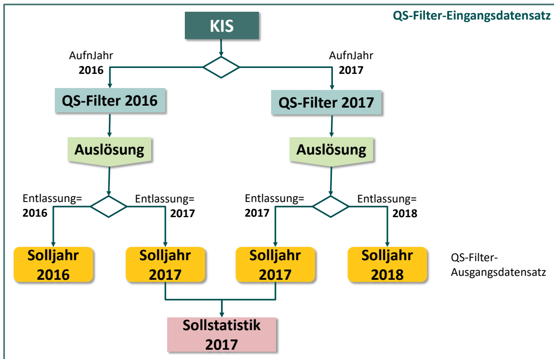
Abbildung 8: Vorgehensweise beim Erstellen der Sollstatistik für lange Überliegerverfahren
