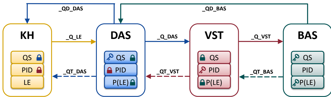
Abbildung 12: Übersicht über die einzusetzenden Suffixe
