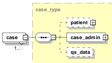
Abbildung 53: Aufbau des Elements case
