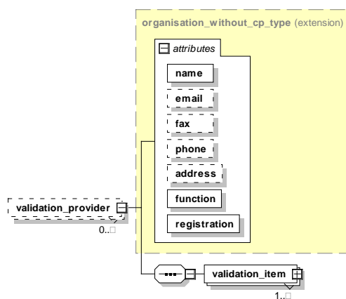
Abbildung 40: Aufbau und Kind-Elemente des Elements validation_provider
