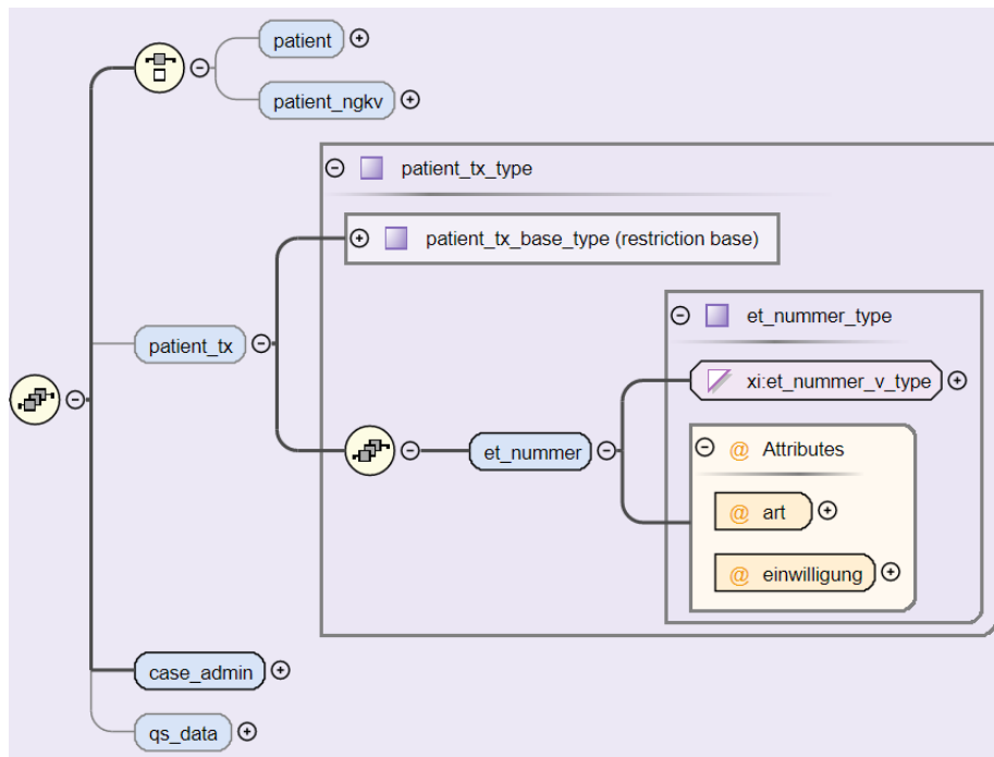
Abbildung 51: Aufbau des Elements patient_tx
