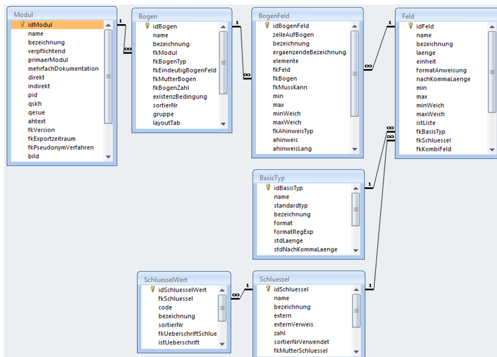
Abbildung 15: Tabellen und Relationen der Datenfelddescription (Beispiel Spezifikation 2017)
