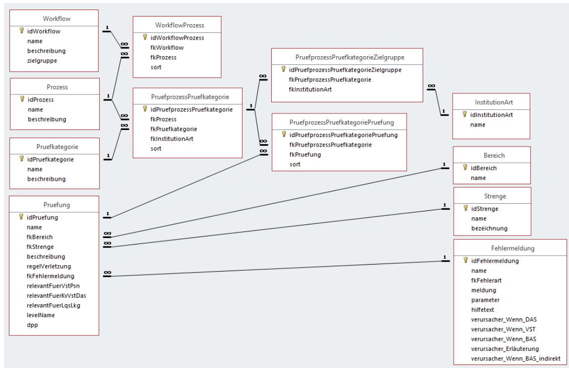
Abbildung 25: Beziehungen der administrativen Objekte – Prüfungen
