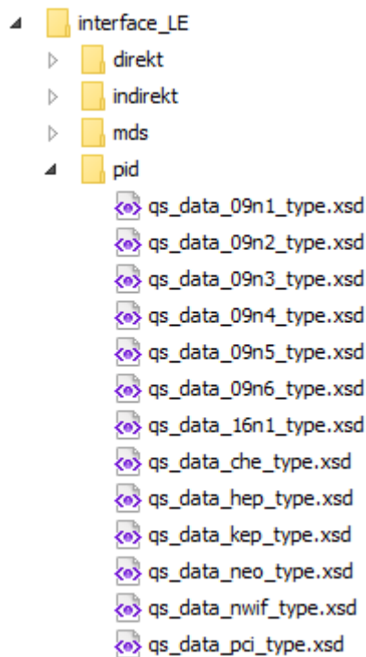
Abbildung 58: Ausprägungen des qs_data -Elements (Erfassungsmodule)
