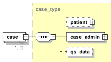
Abbildung 46: Aufbau des Elements case
