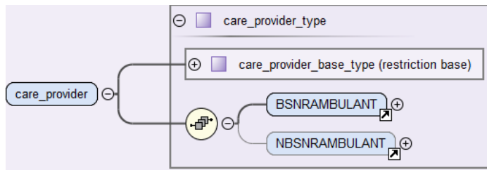
Abbildung 43: Aufbau des Elements care_provider – kollektiv-, selektivvertraglich
