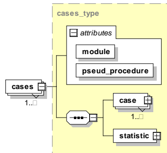
Abbildung 45: Aufbau des Elements cases
