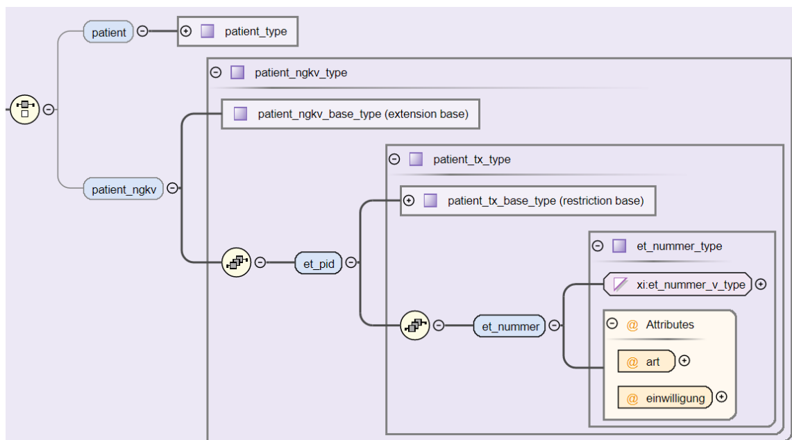
Abbildung 50: Aufbau des Elements patient_ngkv
