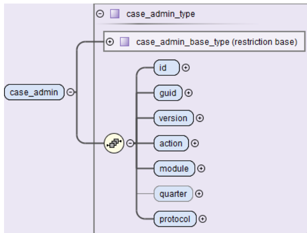
Abbildung 47: Aufbau des Elements case_admin
