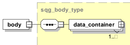
Abbildung 41: Aufbau des Elements body
