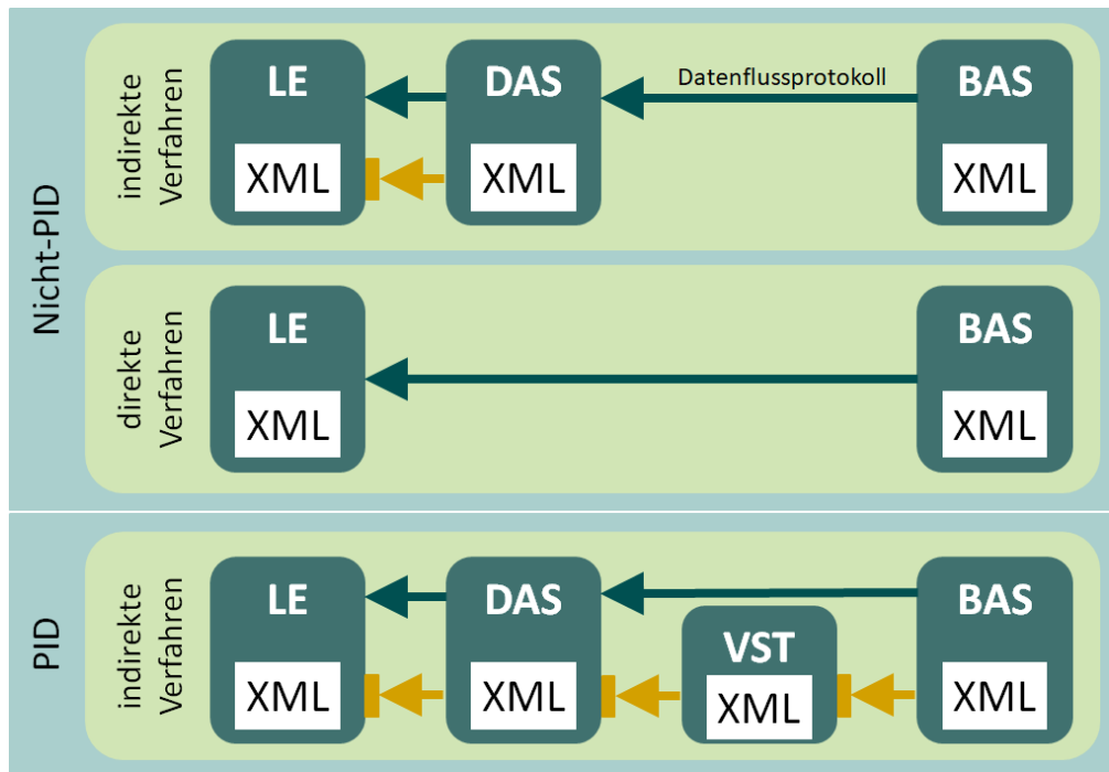
Abbildung 12: Übersicht der Datenflüsse der Rückprotokollierung (orange = Empfangsbestätigung)
