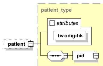
Abbildung 48: Aufbau des Elements patient
