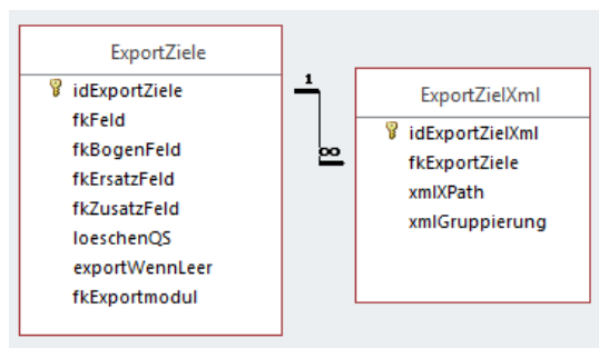
Abbildung 20: Beziehungen der administrativen Objekte – Mapping-Informationen
