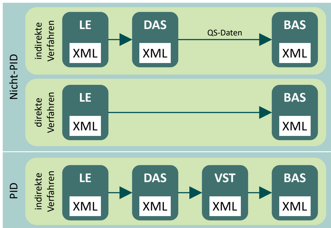
Abbildung 11: Übersicht der Datenflüsse direkte/indirekte PID-/Nicht-PID-Verfahren
