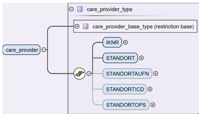
Abbildung 43: Aufbau des Elements care_provider – kollektiv-, selektivvertraglich
