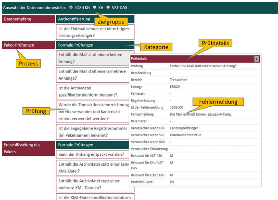
Abbildung 26: HTML-Ansicht der Prüfschritte innerhalb der QS-Dokumentation
